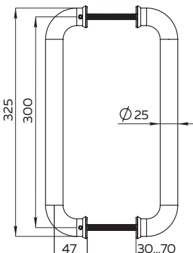
PULL.PH25/200.21 INOX 304
