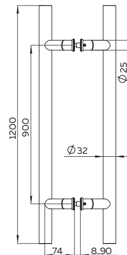
PULL.PH32/1200.45 INOX 304
